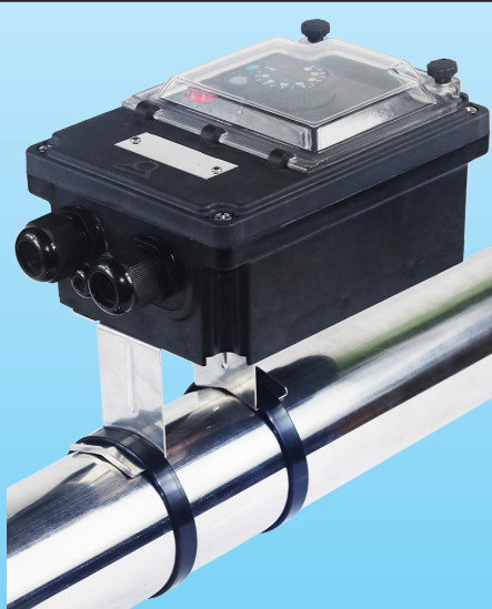
Ejemplo de montaje con la opción de soporte de montaje en la parte trasera 6YTPT en tubería vertical
