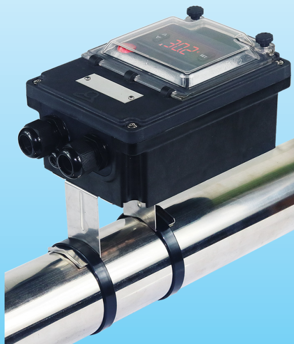
Ejemplo de montaje con soporte de montaje en la parte trasera en tubería vertical
