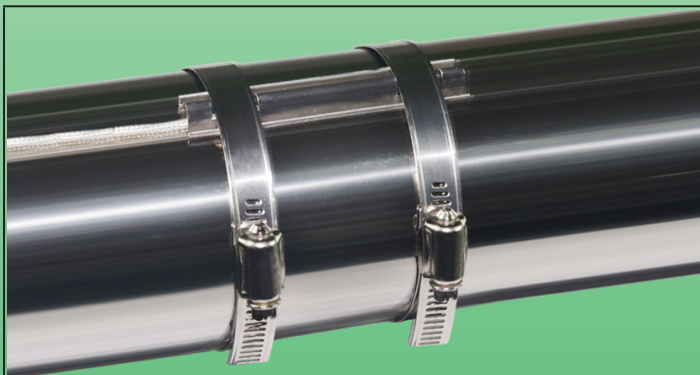
Ejemplo del modelo de sensor de temperatura después de la instalación.
